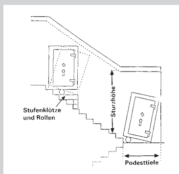
6. Treppe 180° abgewinkelt mit Podest
