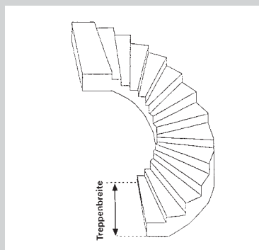
4. Wendeltreppe 180° gebogen
