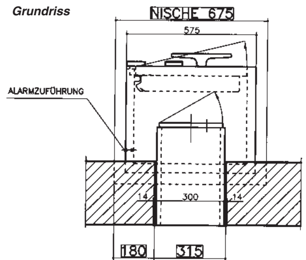
Höhenschnitt und Grundriss (Einwurftresor in Mauer) Beispiel: Mechanischer Einwurftresor LNN 846 Aufnahmeschrank CWH 800
